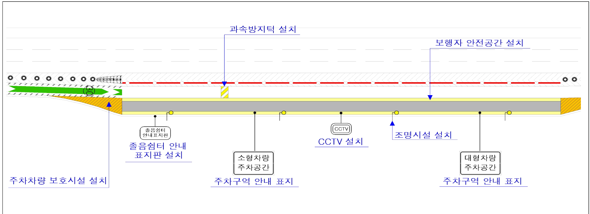
[별표 7] 주행로 및 졸음쉼터 내 안전시설 종류 및 설치 위치
